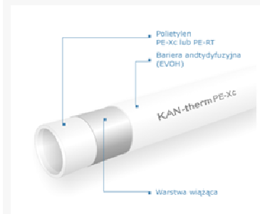
Konstrukcja rur PE-RT lub PE-Xc KAN-therm
